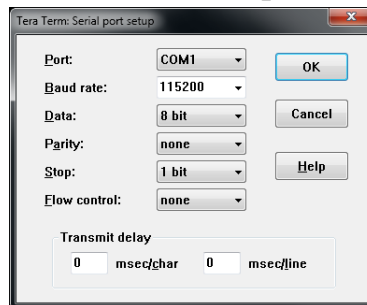
Рисунок 2 - Установка соединения для записи ПО контроллера Compact RTU на процессорный модуль
